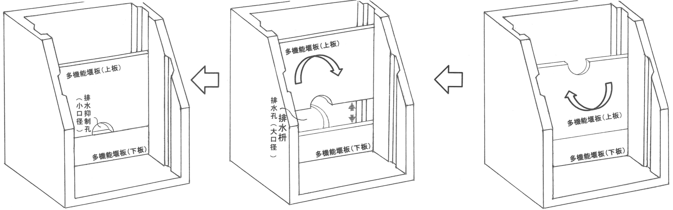
【図2】 排水柵に多機能堰板を設置した側面図 (田んぼダム機能発揮時/図1③)
