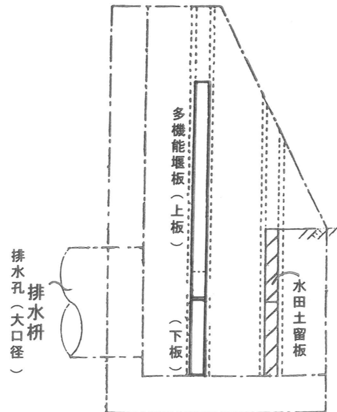
【図2】 排水柵に多機能堰板を設置した側面図 (田んぼダム機能発揮時/図1③)
